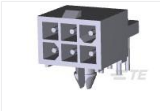
TE Part #1-770969-1 06P MINI UMN L R/A HDR ASSY LF
