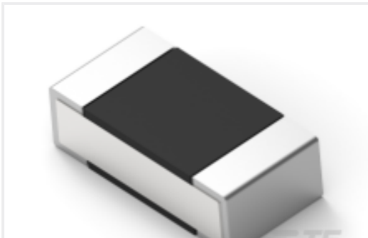
TE Part #2176308-2 RP 1E 0.1W 137K 0.1% 25PPM 5K RL
