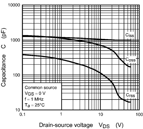
Fig. 8.8 Capacitance - V_{DS}
