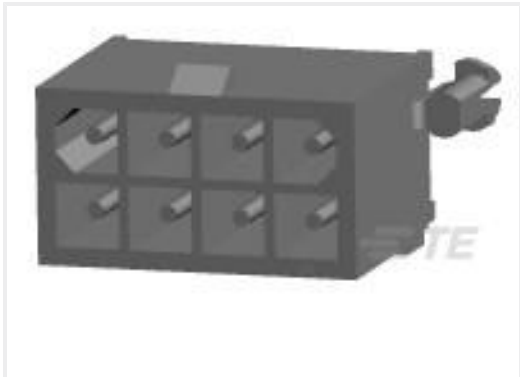
TE Part #1-794065-1 08P MINI UMNL HDR W/DH AU LF
