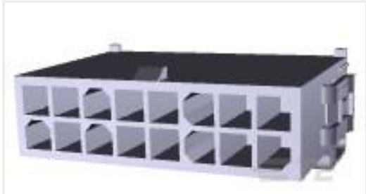
TE Part #794260-1 16P MINI UMNL2 CAP HSG UL94V2
