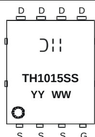
PowerDI5060-8
