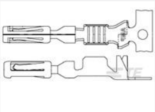
TE Part #770520-3 AMPSEAL,TERMINAL,GOLD PLATE, 16-20AWG WIR
